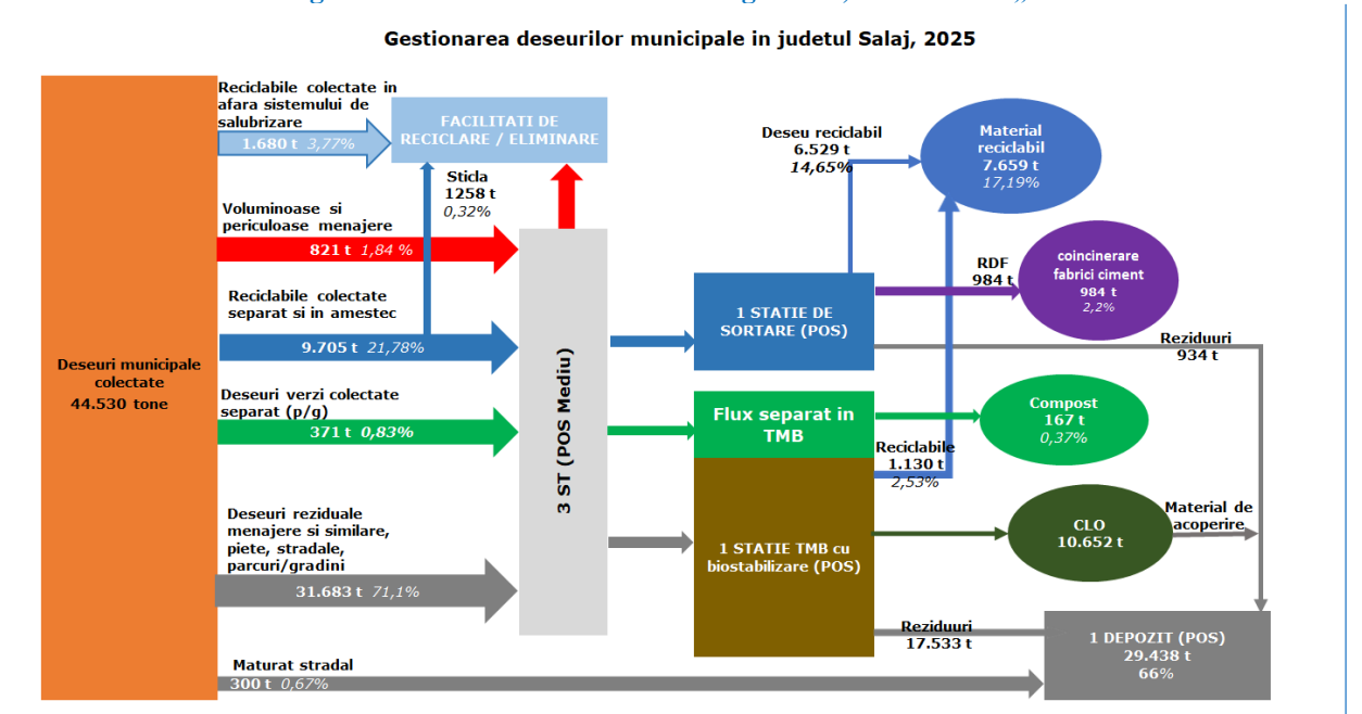
Figura 7-22 Schema fluxului tehnologic 2025, Alternativă „zero”
